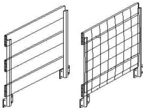
Fig. 1 – Parapetto con corrente intermedio e parapetto con protezione intermedia costituita da una rete di tipo U (immagine tratta da ISPESL, Linee guida per la scelta, l'uso e la manutenzione dei sistemi collettivi di protezione dei bordi).
